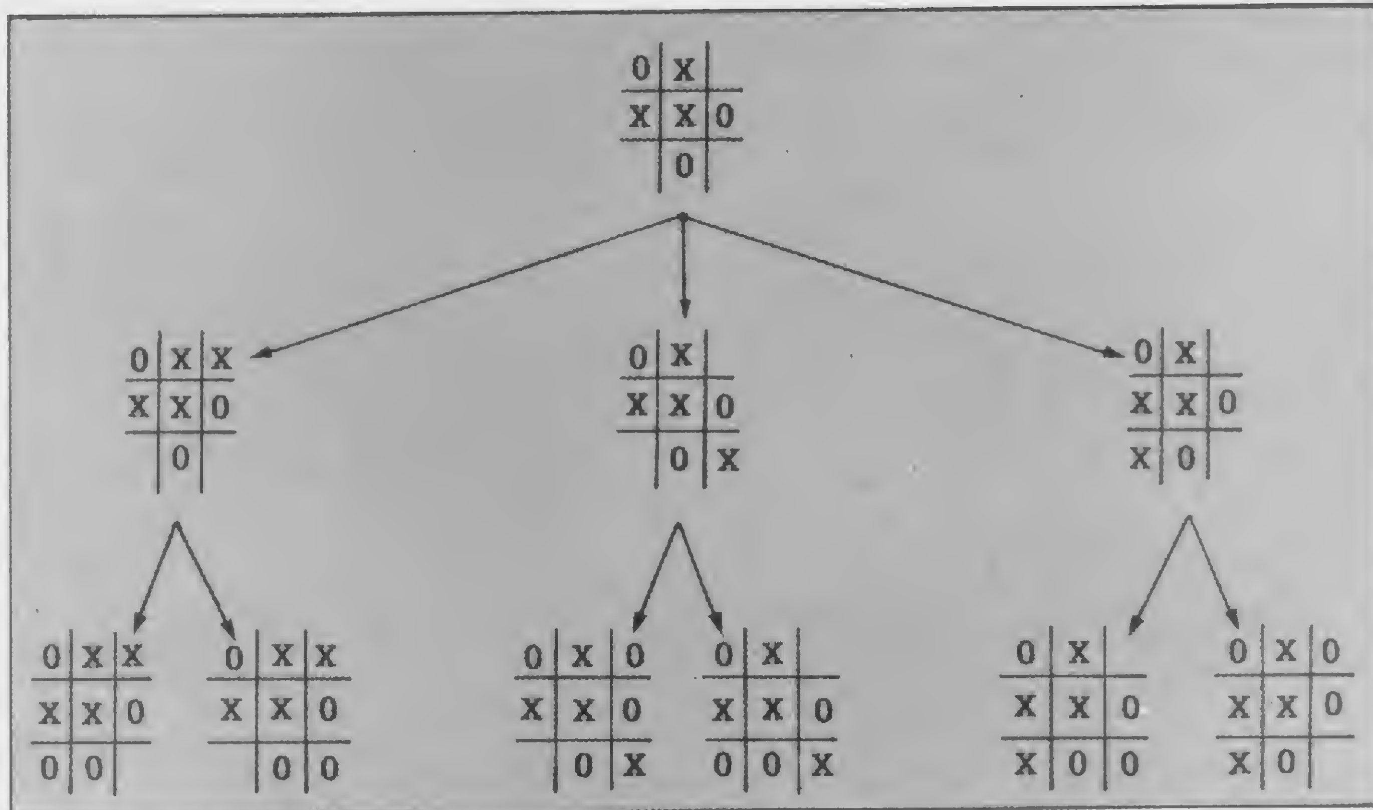
Figura 4 - Os lances possíveis de X, seguidos dos lances possíveis de 0
